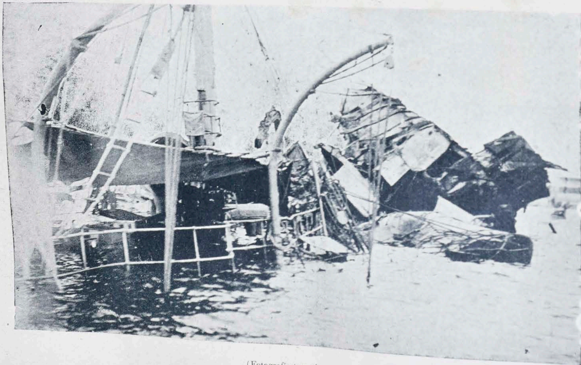
(Fotografía tomada expresamente para EL FIGARO, por el Sr. Gómez Carrera) Puente del Maine , visto por el lado de babor.
